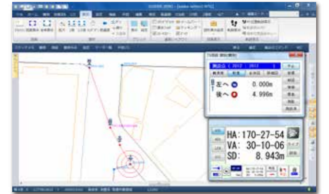
GUIDER ZERO測設画面
