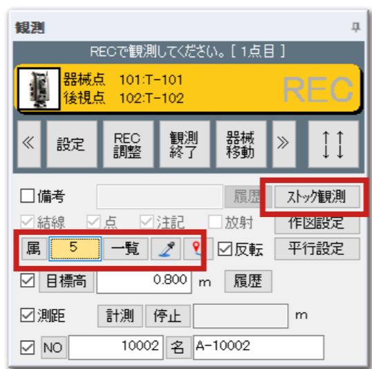
TS観測による「属性観測」
